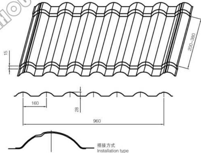
立体效果图 Stereo view
