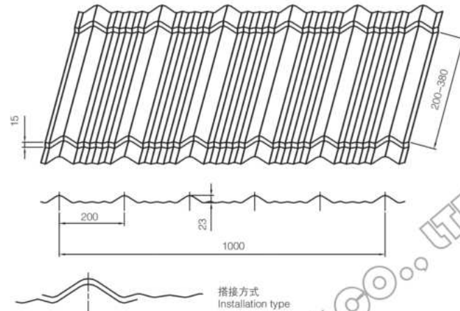
立体效果图 Stereo view
