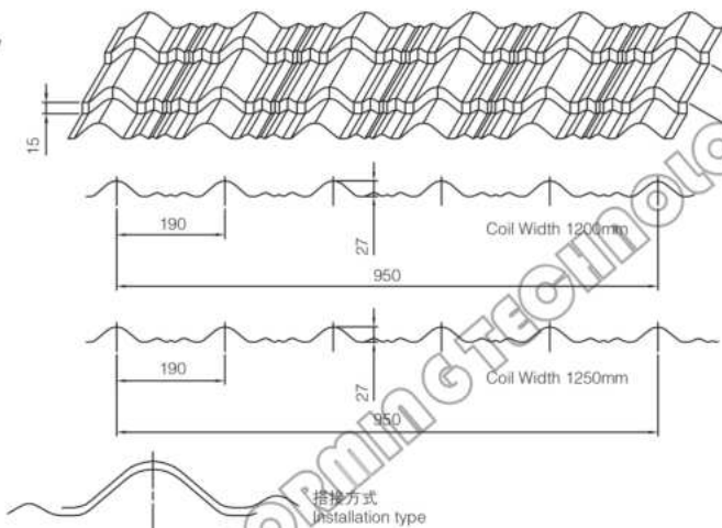
立体效果图 Stereo view
