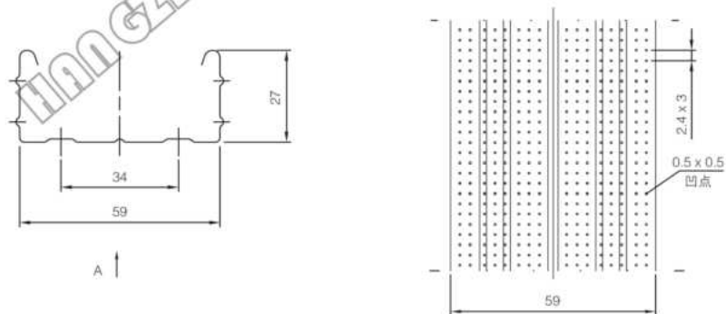
A向 底面压花图 Embossing drawings
