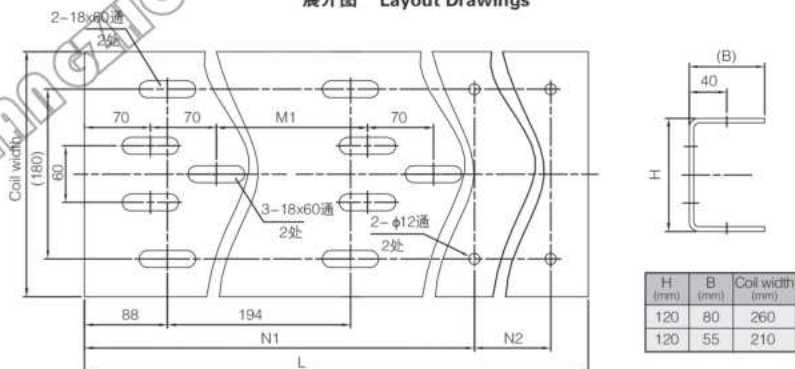
展开图 Layout Drawings
