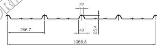
搭接方式 Installation type
