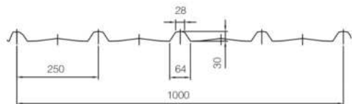
搭接方式 Installation type
