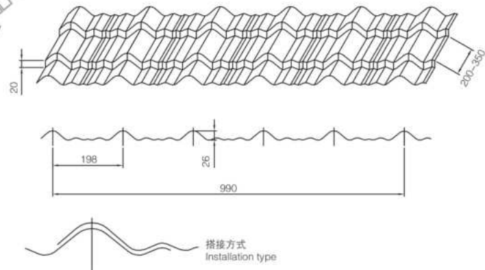
立体效果图 Stereo view
