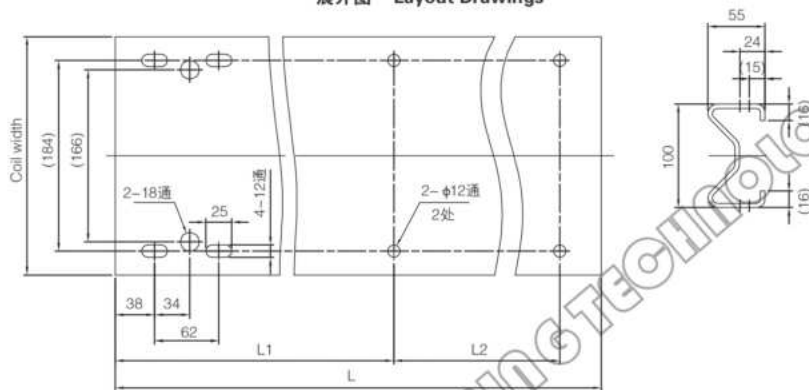
展开图 Layout Drawings
